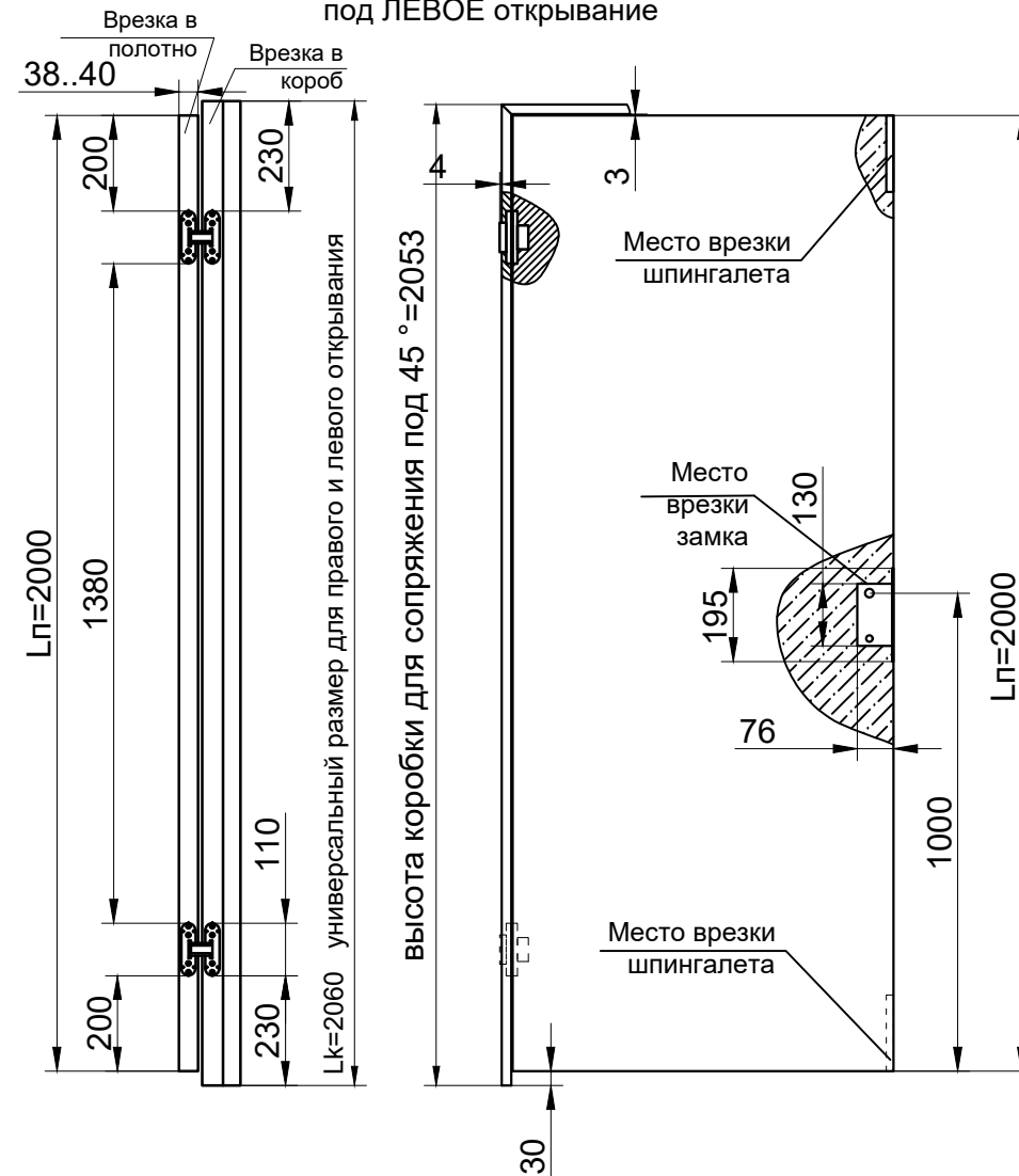
Схема резки петли НН -24 под ЛЕВОЕ открывание
