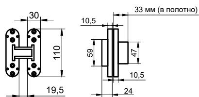
Петля НН-24
