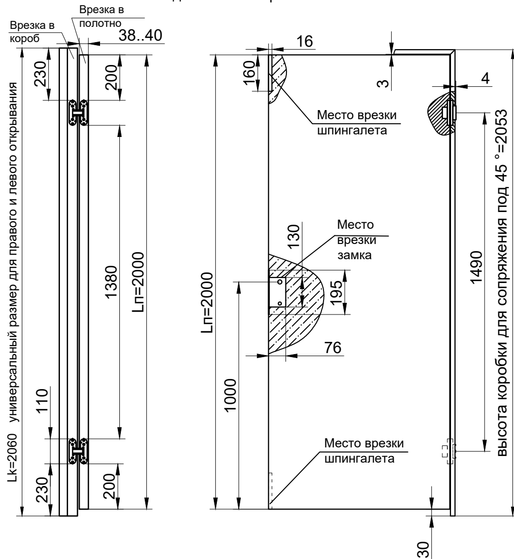
Петля НН-24
