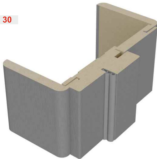
Т-телескопический погонаж
